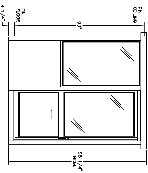
ELEVATION A
